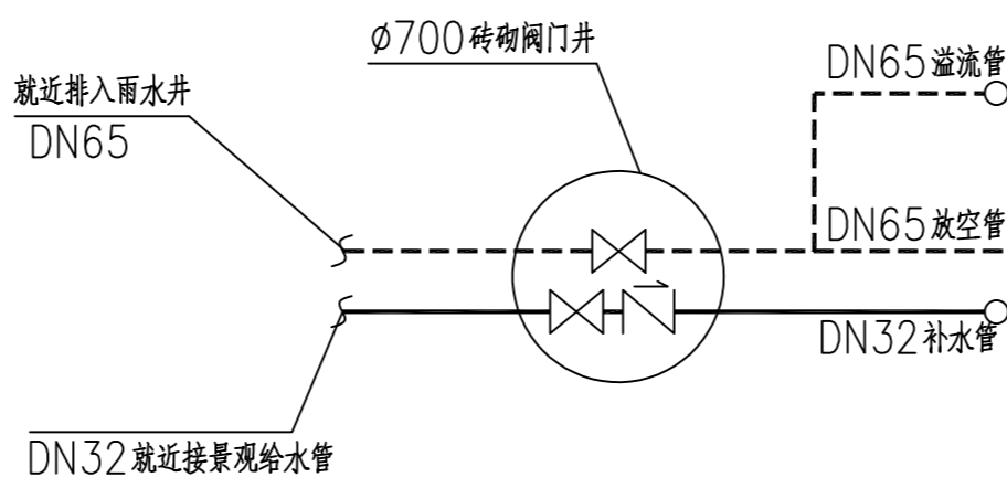
景观给排水管道平面图
