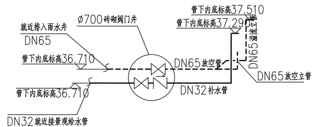
景观给排水管道系统图
